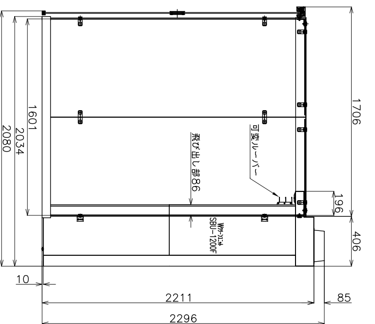
SmokingRoom 側面図
