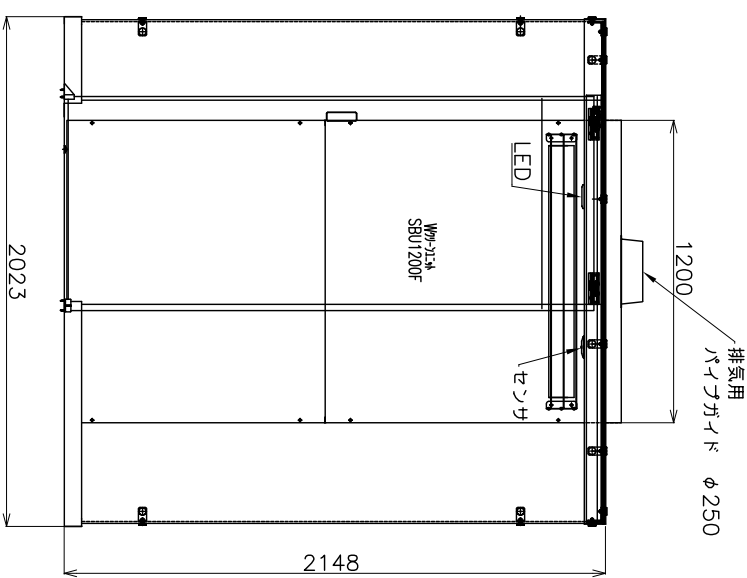
SmokingRoom正面図
