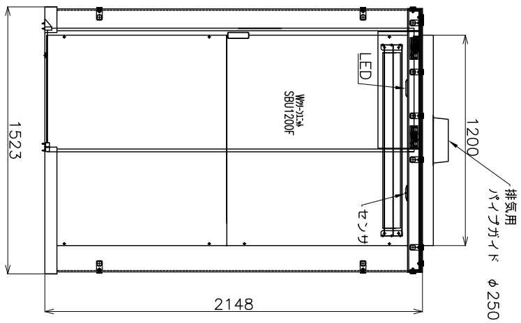
SmokingRoom正面图
