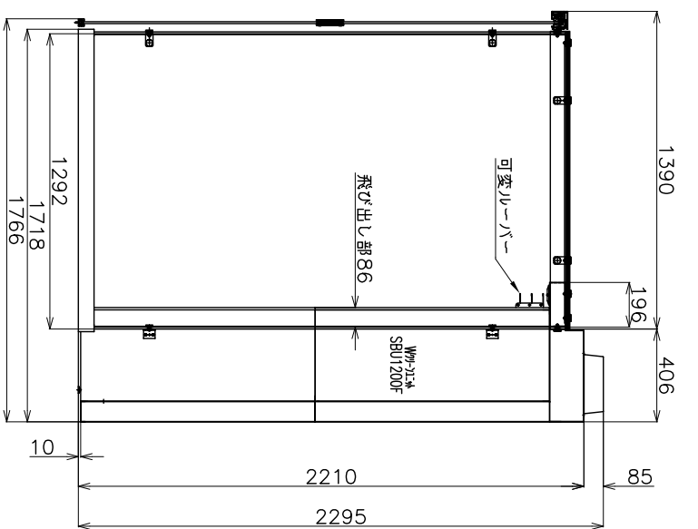
SmokingRoom 側面図
